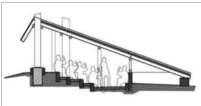
SYSTEMSCHNITT A-A
